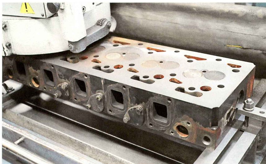
Planschleifen und Fräsen von Zylinderköpfen bietet Derendinger als Dienstleistung ebenfalls an. Fotos: Derendinger
